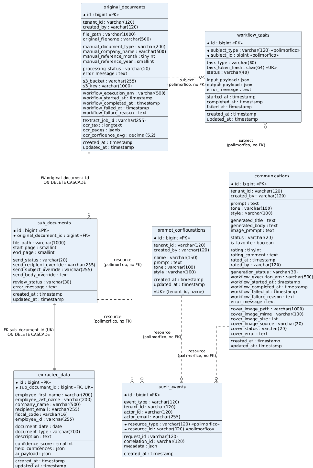
Figura 127: Schema ERD
